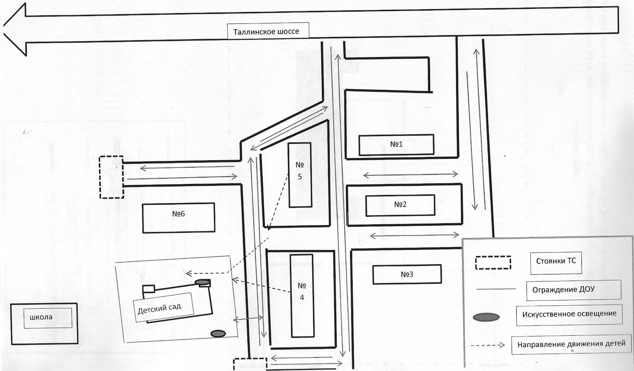
2. Схема организации дорожного движения в непосредственной близости от образовательного учреждения с размещением соответствующих технических средств, маршруты движения детей и расположение парковочных мест
